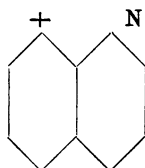
Schöllkopf.
